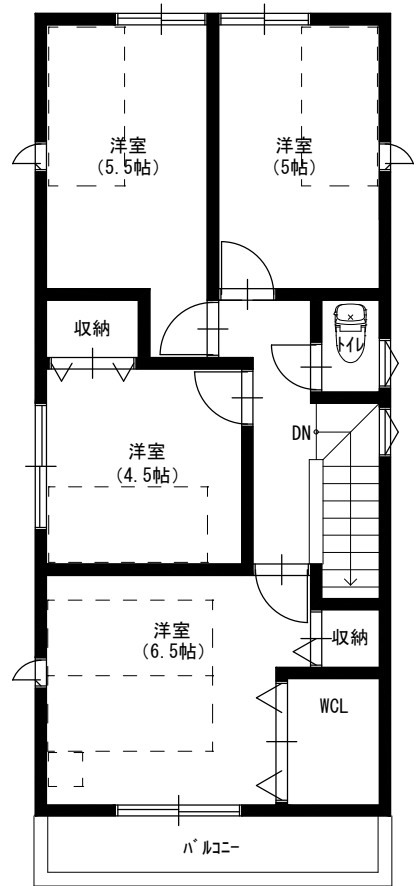
2階 平面図 S:1/100
